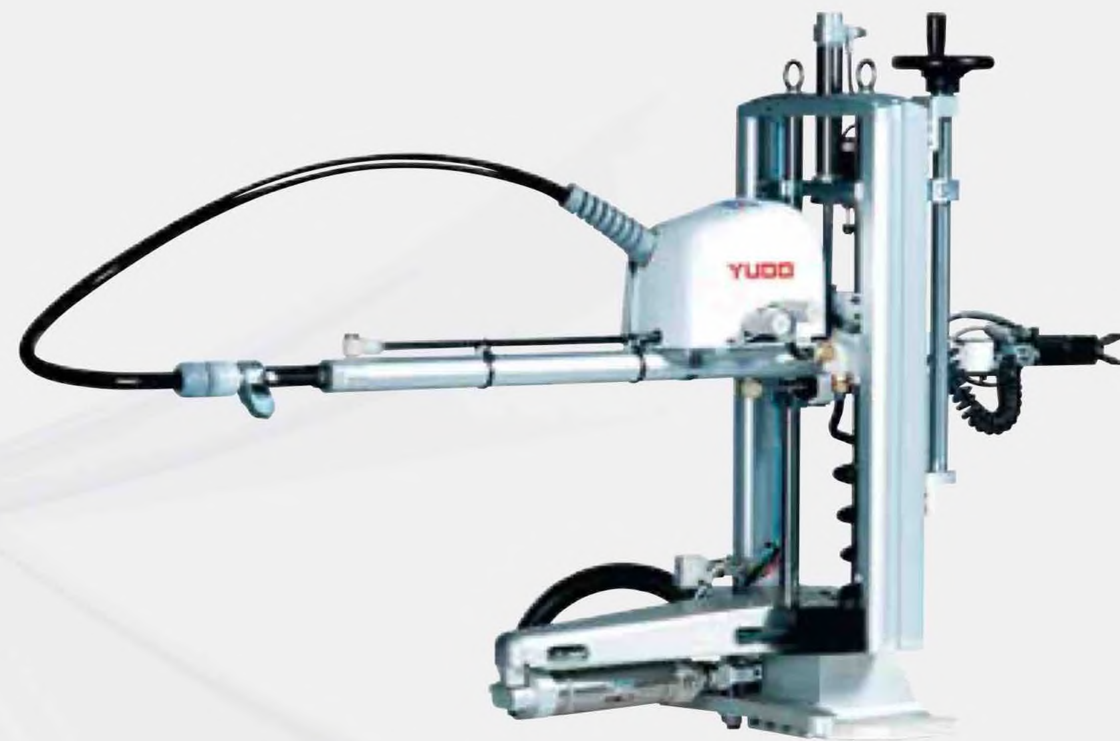
다대 사출기 대응의 SMUS-600FH Side entry type
